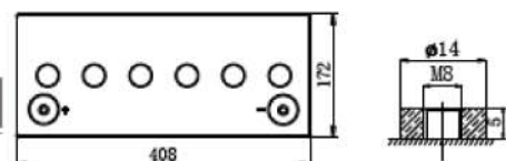
Вывод В-М8
