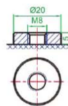
Вывод В-M8
