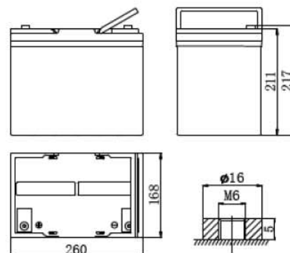
Вывод В-M6
