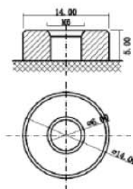
Вывод В-М6
