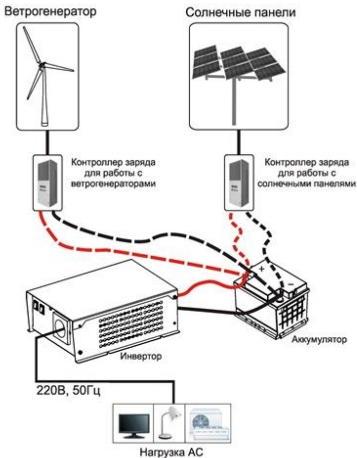
Рисунок 3. Схема подключения инверторов серии СибВатт к системам альтернативной энергетики
