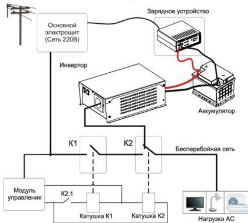
Рисунок 2. Схема подключения инверторов серии СибВатт к системам бесперебойного питания
