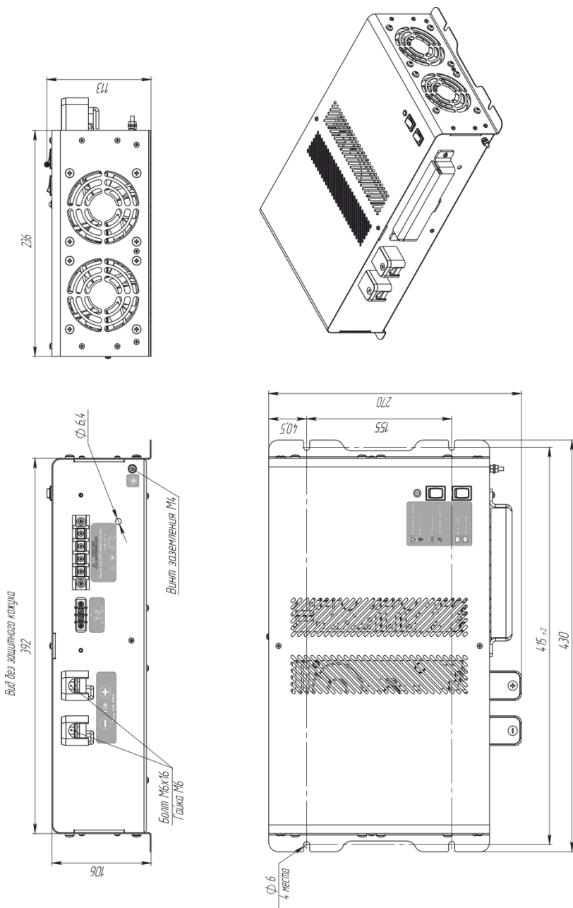
Рис. 1-б Внешний вид СибВатт 3512/4024
