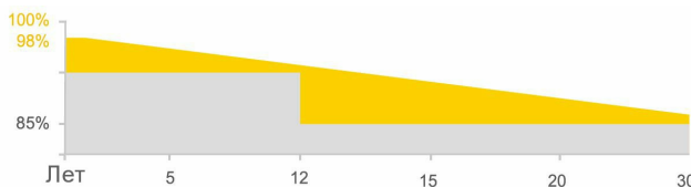
Прогнозируемое сохранение мощности солнечного модуля
