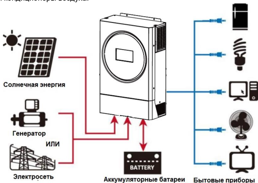
Рисунок 1. Структурная схема подключения гибридной солнечной электростанции
